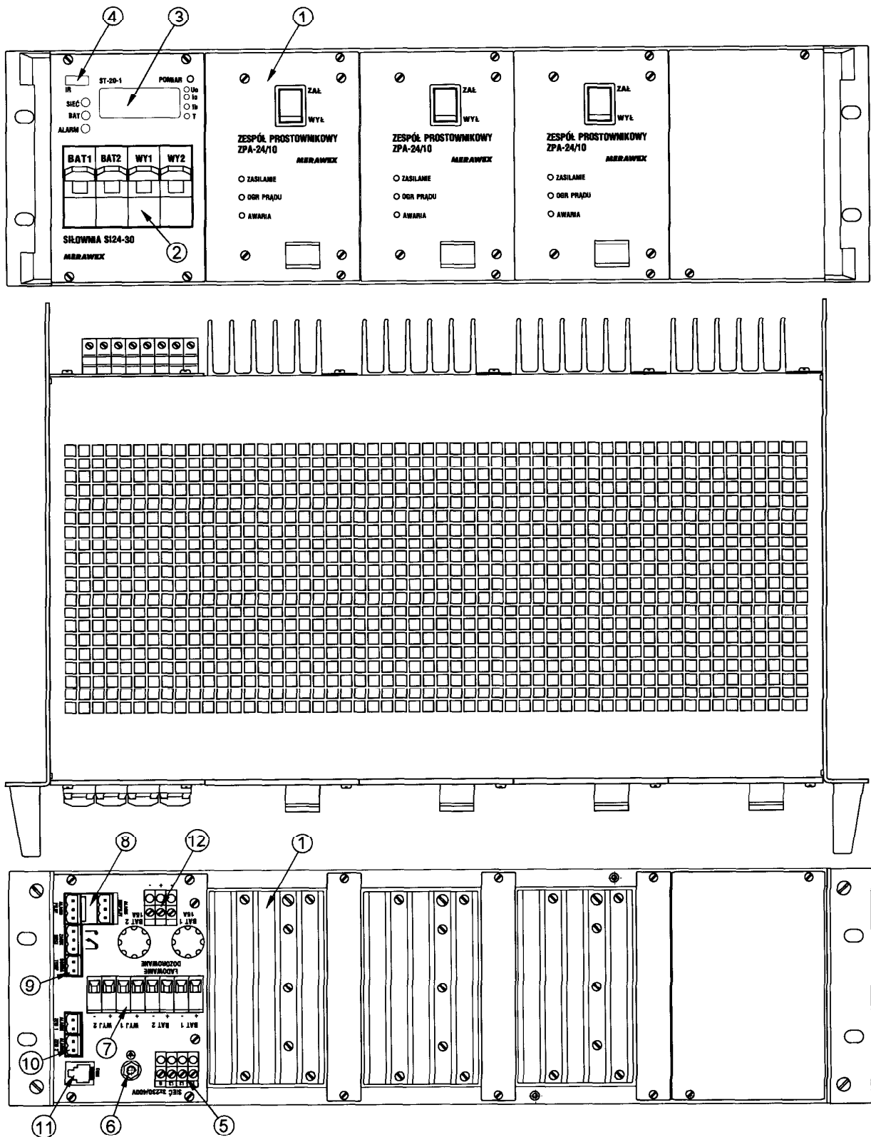
Rys.2. Wygląd zewnętrzny siłowni SI24-30-31 (urządzenie w pełnej konfiguracji – zawiera opcjonalne wejście zewnętrzne obwodu ładowania dozorowanego).
