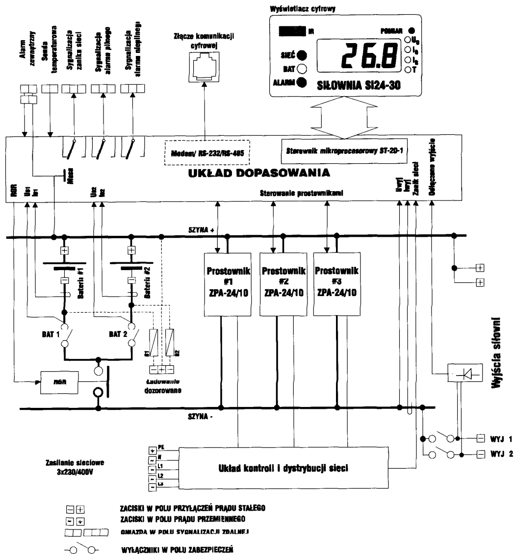
Rys. 3. Schemat blokowy siłowni SI24-30-31
