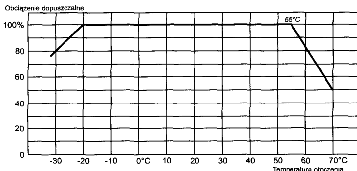
Rys.1 Dopuszczalne obciążenie siłowni w funkcji temperatury otoczenia
