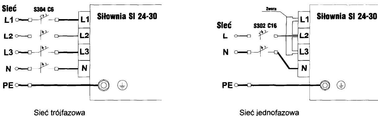
Rys.5 Schemat podłączenia zasilania siłowni SI24-30.
